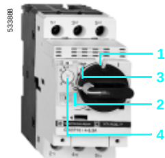
GV2 P
